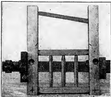
Fig. 229—Clamping Taboret
